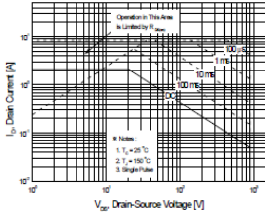
图 6-2 最大安全工作区曲线(TO-220F)
